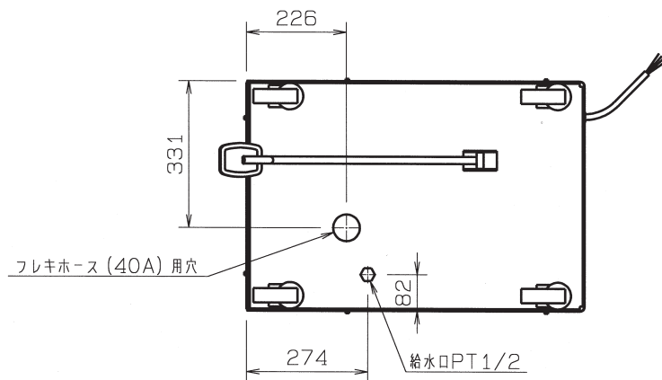
●底面図
