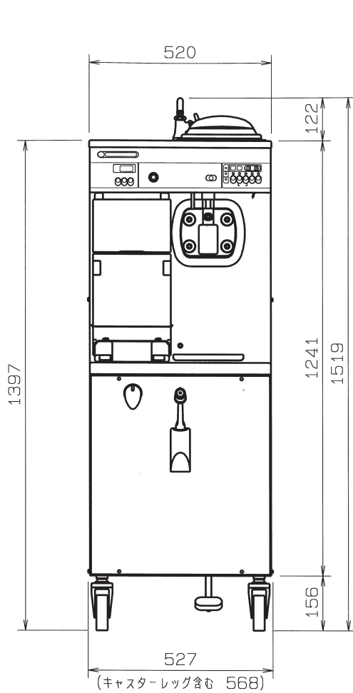
●前面図
