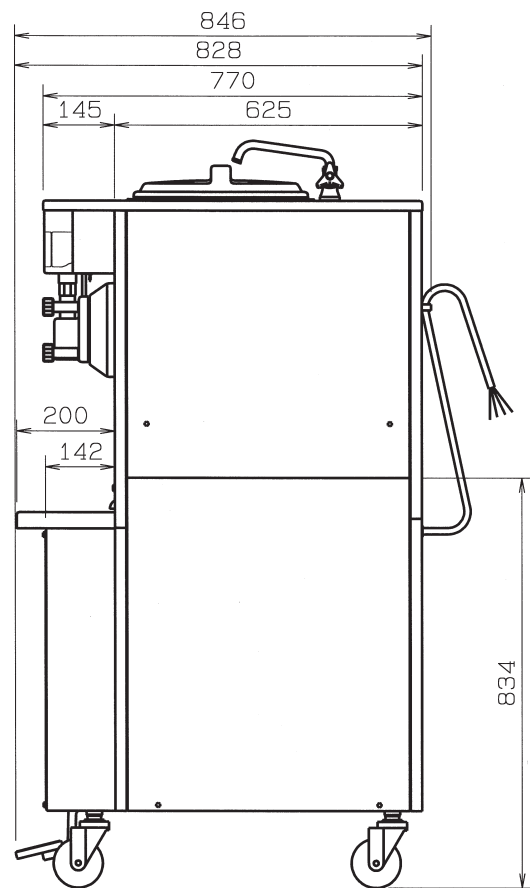
●側面図
