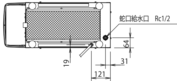
●底面図
