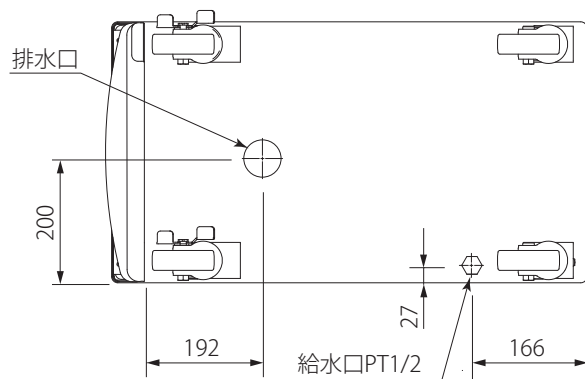
●底面図
